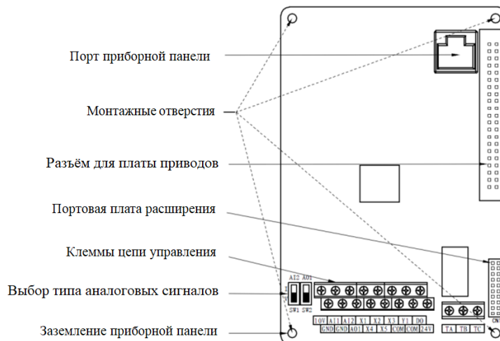
Рис. 3-20 Плата управления
