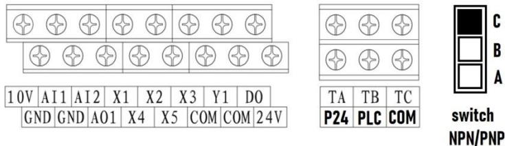
Рис. 3-10 Расположение клемм цепи управления для версии B2_0102
